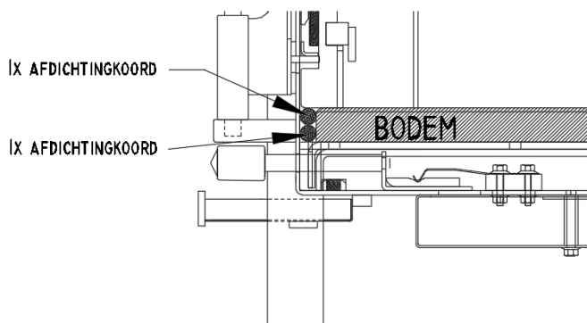
Dwarsdoorsnede brandkamer:
